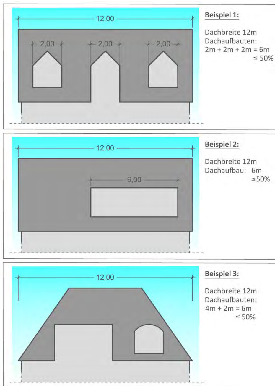
Abbildung Schematische Darstellung der Begrenzung von Dachaufbauten und -einschnitten bei geneigtem Hauptdach (drei Beispiele)
