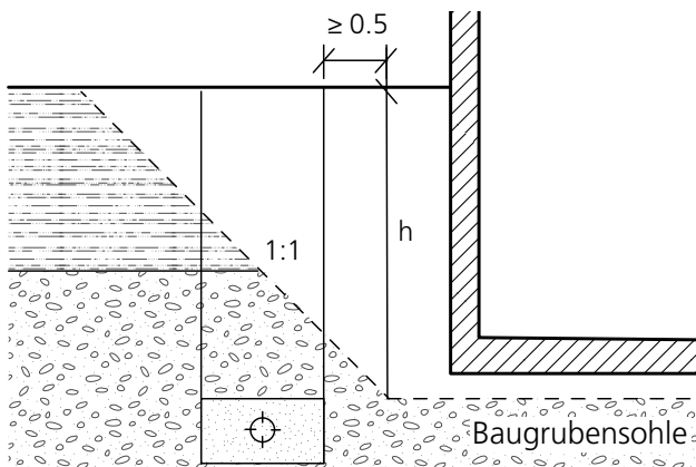
Rigole als Entwässerungsmaßnahme / Querschnitt
