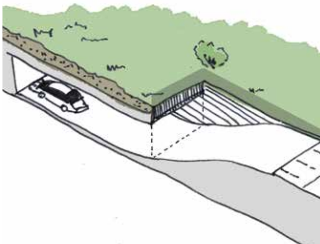
Schemaskizze 'Tiefgarage mit begrüntem Dach'
