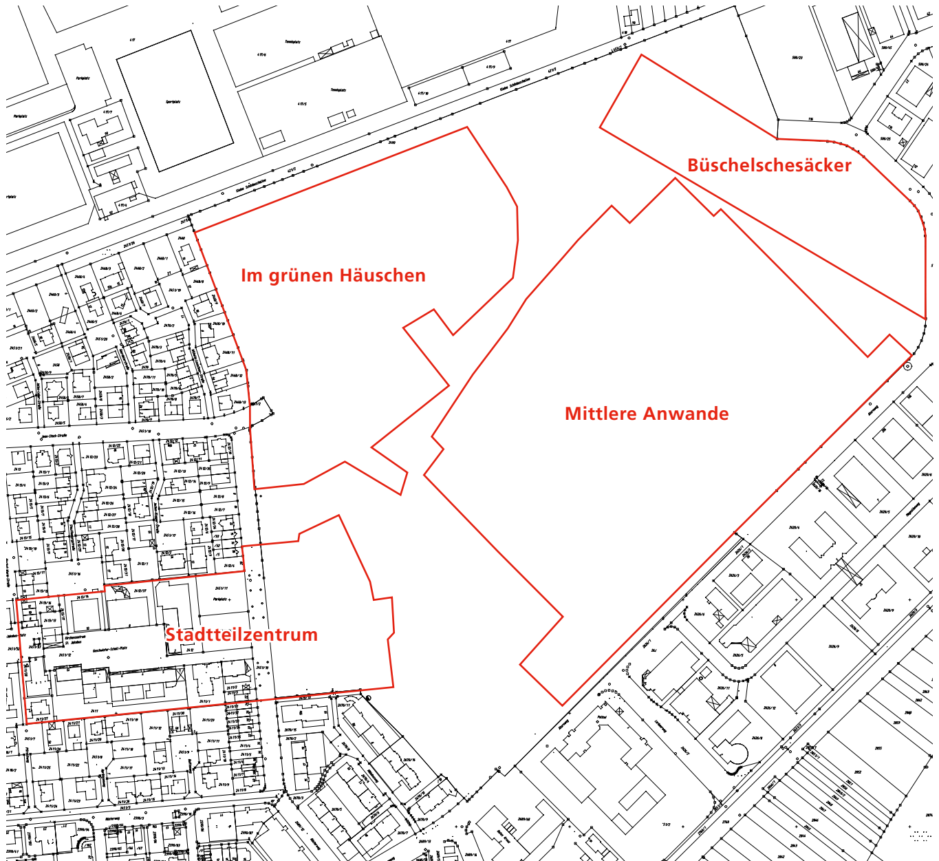
Übersichtsgrafik Teilbaugebiete
