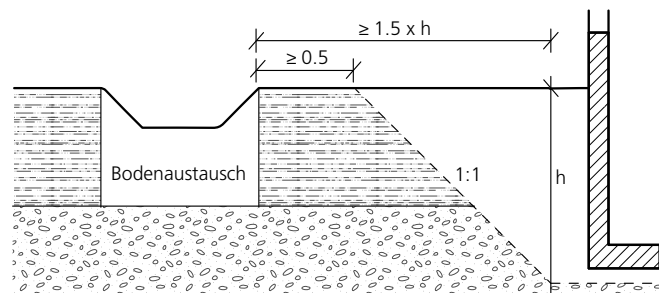
Versickerungsmulde als Entwässerungsmaßnahme
