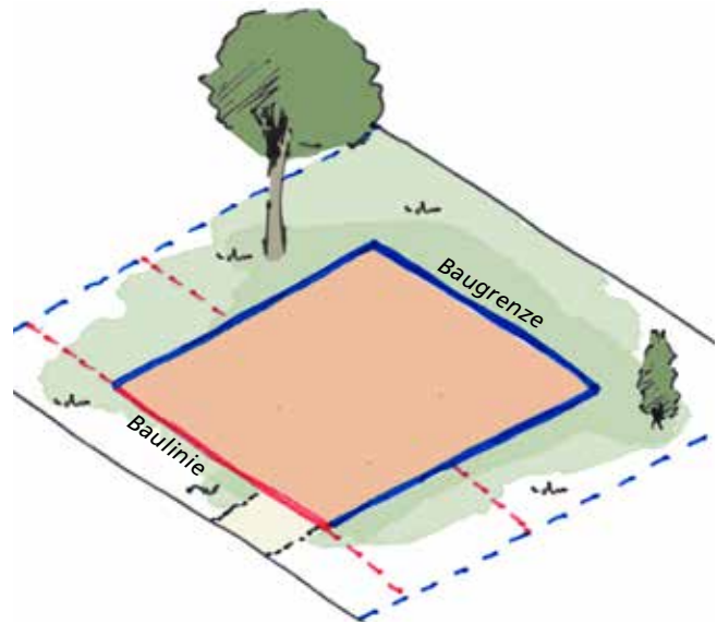
Baugrenzen und Baulinien
