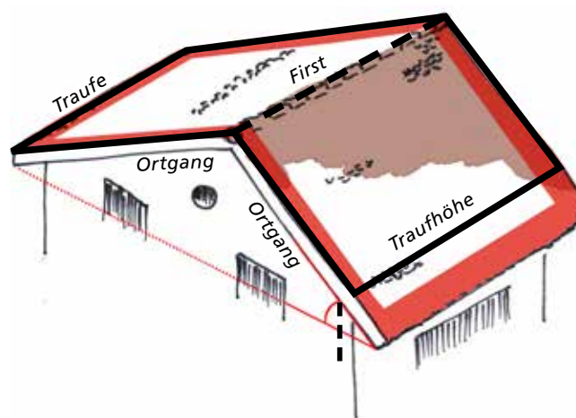
Dachaufbau
