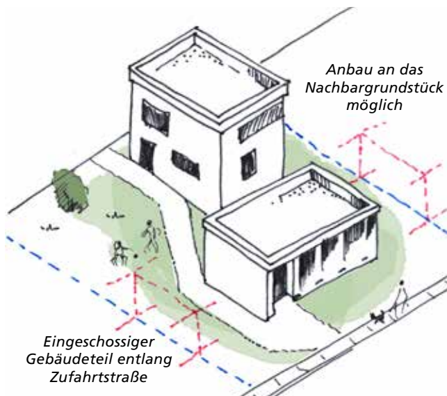
Schemaskizze 'Gebäudetyp WA 8'
