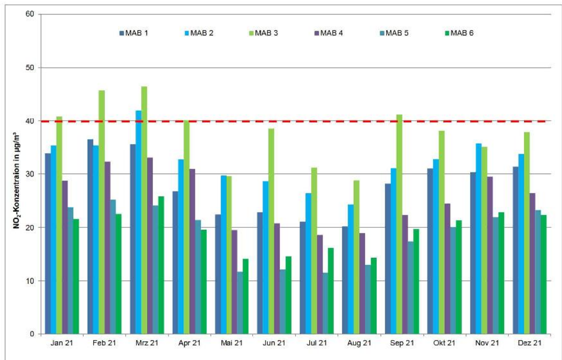
Abbildung 9. Verlauf der gemessenen \text{NO}_2 -Konzentrationen an den Messstandorten MAB-1 bis MAB-6 für den Messzeitraum 04.01.21 - 03.01.22 (Monatsmittelwerte, \text{NO}_2 -Grenzwert für das Kalenderjahr 40 \mu\text{g}/\text{m}^3 rot gestrichelt markiert).
