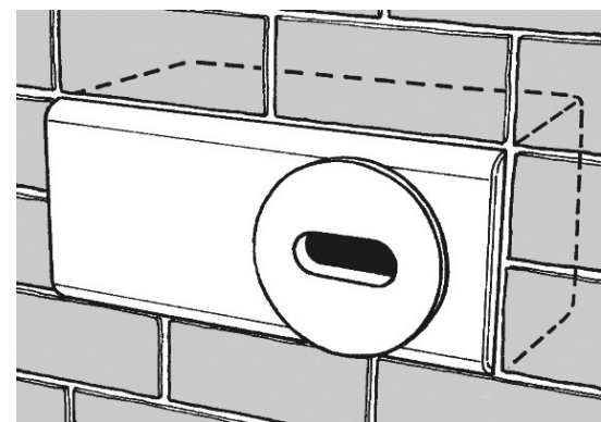
Einbauschema © Schwegler
