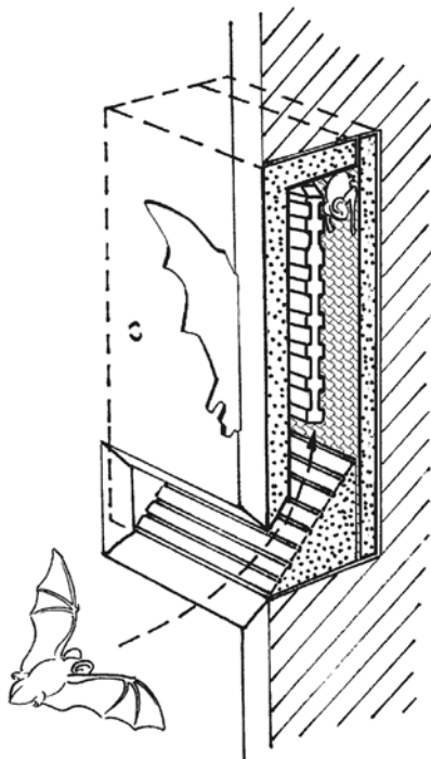
Schnitt Fledermauskasten
